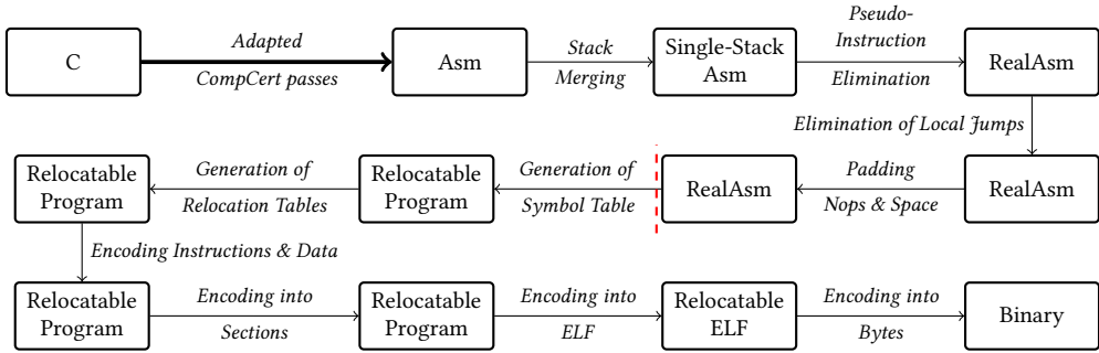
Fig. 9. CompCertELF
